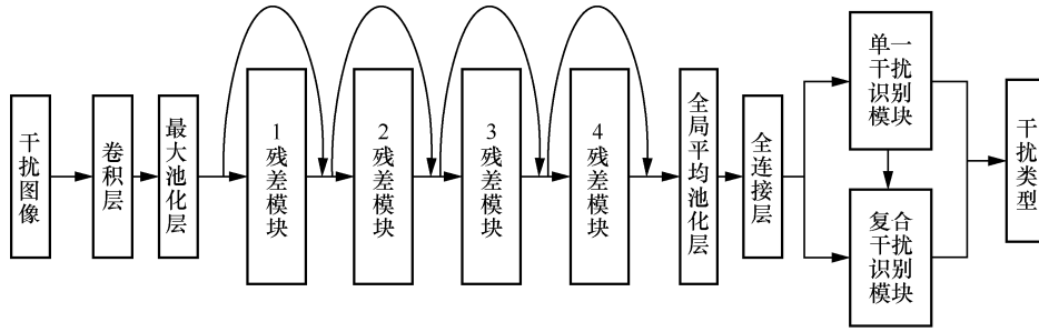
图6 改进残差网络结构
